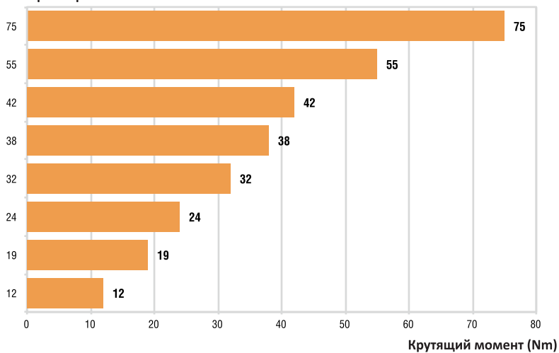
Типоразмер ZL
